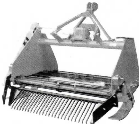
UTD-1052 (ソリ・補助機付)
