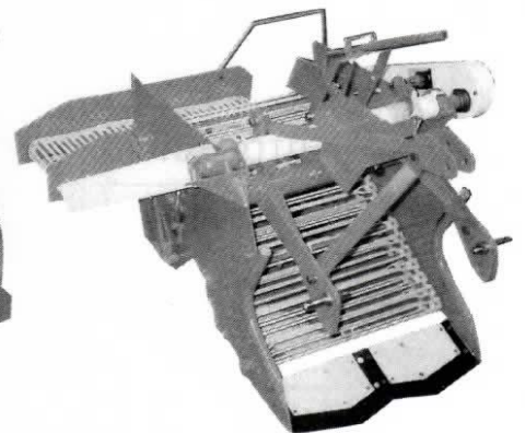
UTD-680LSN (サイドコンベア付)
